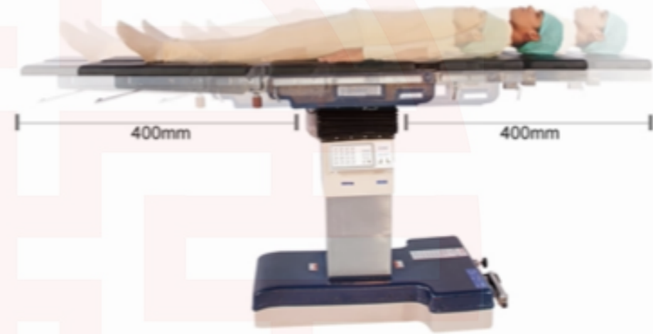
Longitudinal sliding
